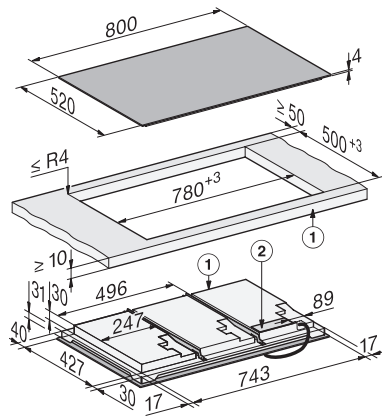
KM8885FL Diamond&MSense, aufliegender Einbau, (*Fußnote) Skizze
