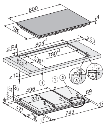
KM8885FL Diamond&MSense, flächenbündig, (*Fußnote) Skizze
