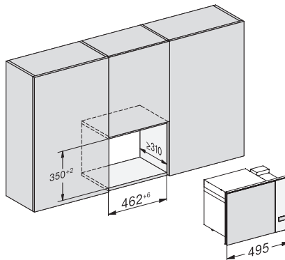
M22xxSC, Skizze
